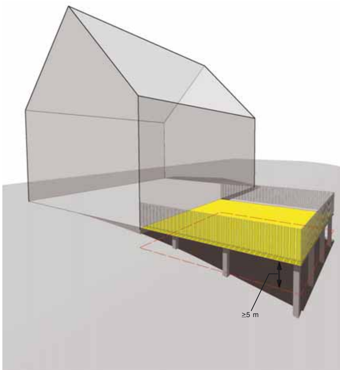
Fig 2-9 Bygningsdeler og konstruksjoner som ligger mer enn 0,5 m over planert terreng gjennomsnittsnivå rundt byggverket skal medregnes i bebygd areal.
