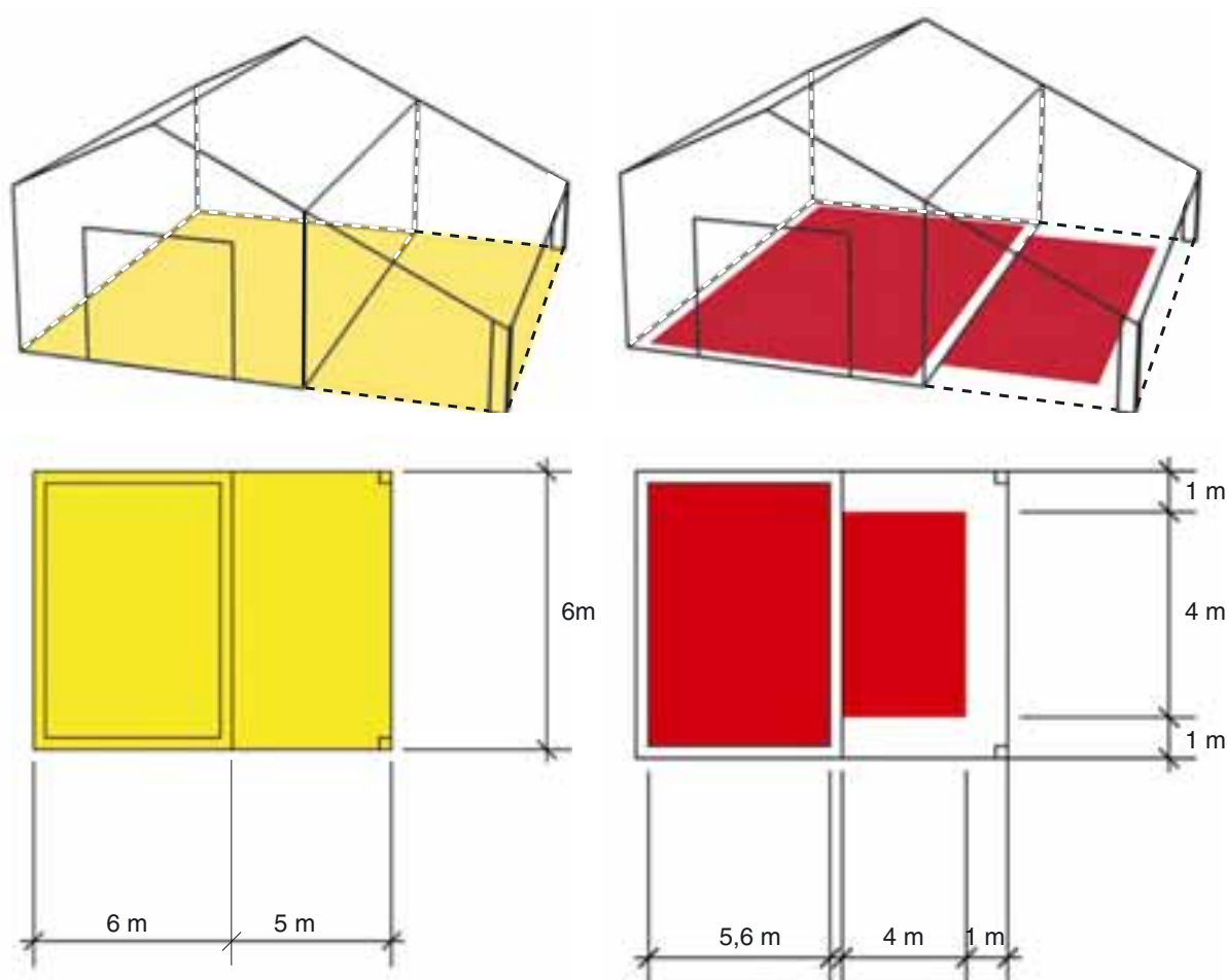
Fig 4-14 Mindre bygning som beskrevet i plan- og bygningsloven § 70 nr. 2 annet ledd bokstav b, er bygning hvor verken samlet bruksareal eller bebygd areal er over 50 m 2
