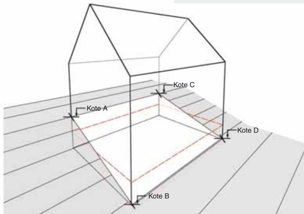
Fig 2-27 Enkel beregning av planert terrengs gjennomsnittsnivå
