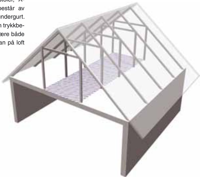
Fig 3-5 Måleverdig golvplan på loft med A-takstol
