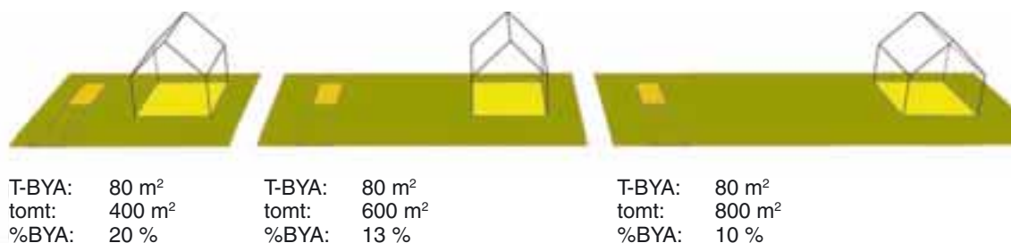
Figur 2-3 Totalt bebygd areal for en tomt egner seg der det ikke er av betydning å fastsette forholdet mellom tomteareal og bygningsvolum, f.eks. i områder for spredt bolig- og fritidsbebyggelse
