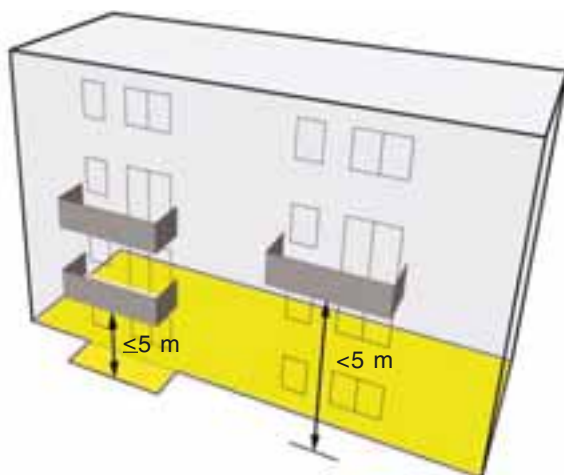
Fig 2-8 Utkragede bygningsdeler medregnes i bebygd areal når høyden til planert terreng er høyst 5,0 m
