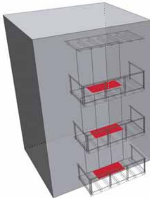
Fig 2-20 Åpent areal under overbygd terrasse og balkonger som ligger mer enn 1,0 m innenfor ytterkant av dekket over skal legges til bruksarealet
