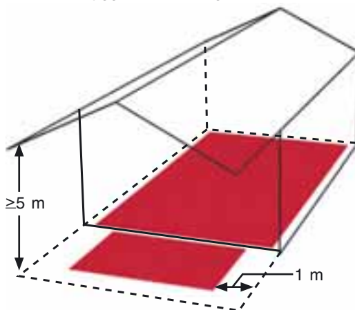
Fig 2-19 Areal under takutstikk som er mer enn 1,0 m innenfor ytterkant av takutstikk, skal legges til bruksarealet
