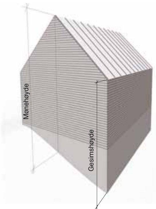
Figur 4-12 Måling av høyde som beskrevet teknisk forskrift § 7-26 nr. 2. Høyde måles fra møne eller gesims langs fasaden loddrett ned til underliggende planert terreng
