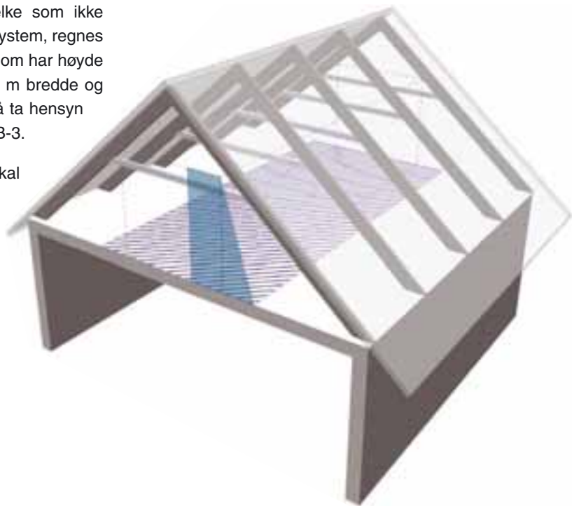
Fig 3-4 Måleverdig golvplan på loft med taksperrer eller hanebjelke som ikke er del av takkonstruksjonens statiske system
