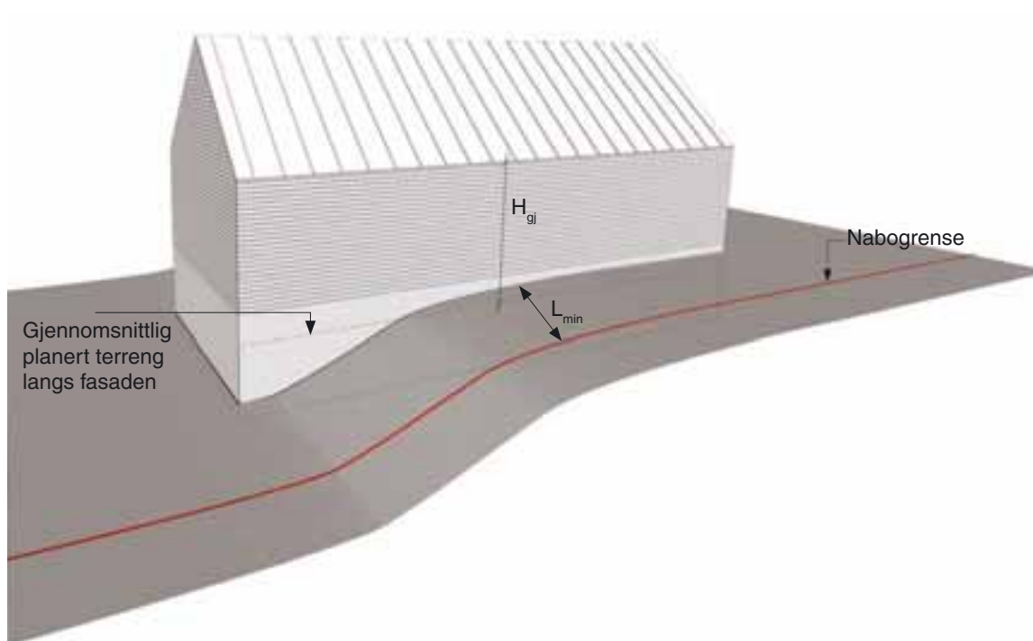
Figur 4-11 Måling av gesimshøyde som beskrevet i plan- og bygningsloven § 70 nr. 2
