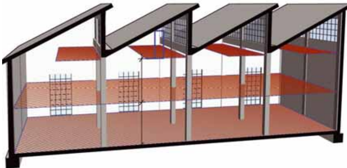
Fig 2-22 Areal i rom med høyde 4,9 m eller mer, måles med tenkte plan for hver 3,0 m høyde. På figuren medregnes det som er markert med raster
