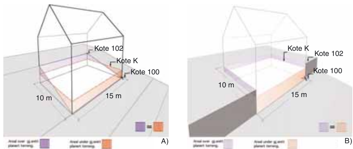
Fig 2-28 Gjennomsnittlig planert terreng i eksempel A) og B)
