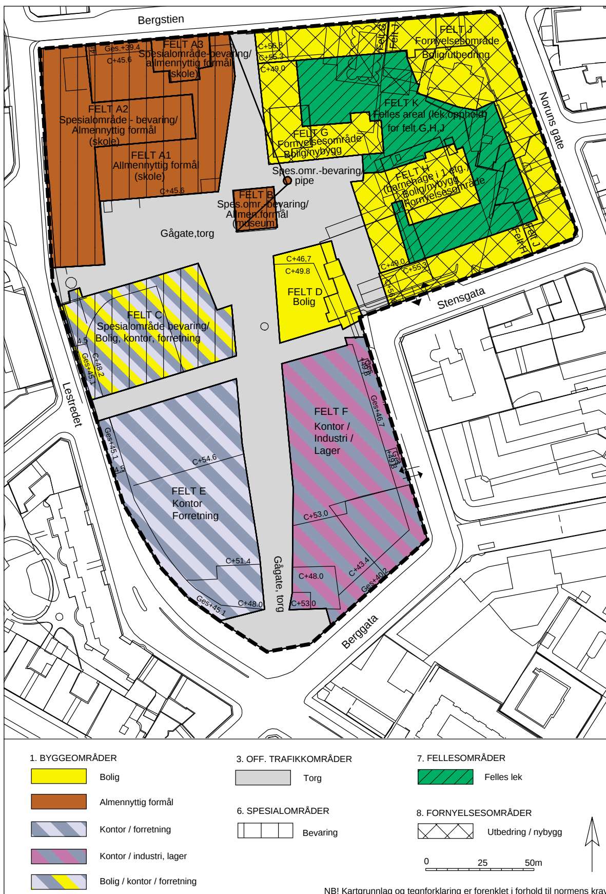
Figur 3.12. Reguleringsplan med tilhørende bestemmelser for mer sammensatt og krevende by-/ tettstedssituasjon med krav om nærmere detaljering / bebyggelsesplan i reguleringsbestemmelsene. Eksemplet viser både eksisterende og nytt, blandede formål, bevaring og fornyelsesområde
