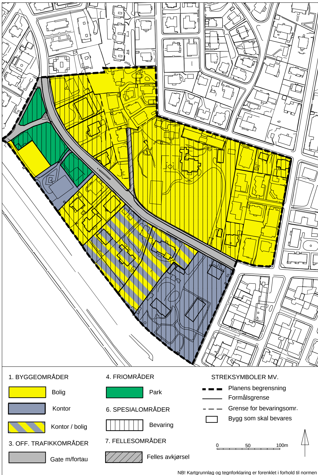
Figur 3.20. Reguleringsplan med bestemmelser som viser bygninger og anlegg som på grunn av historisk, antikvarisk eller annen kulturell verdi skal bevares.
