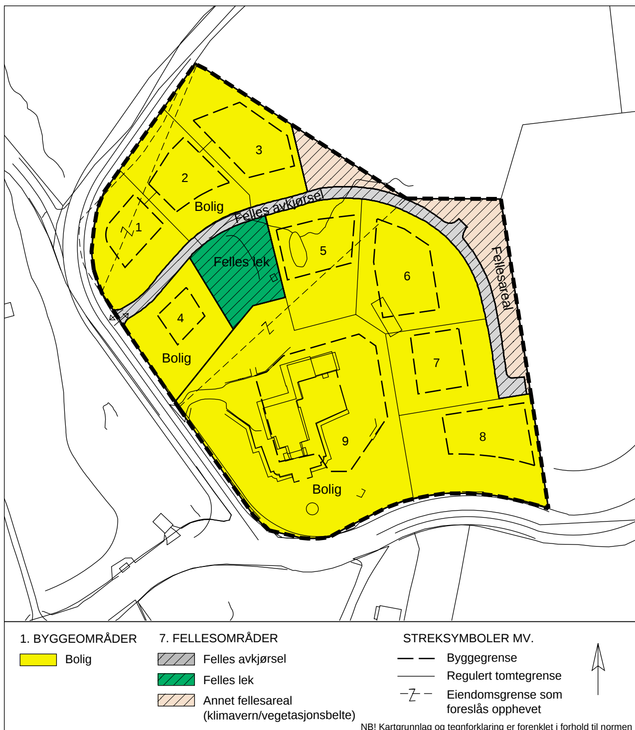
Figur 3.16. Bebyggelsesplan for mindre boligområde etter krav i kommuneplan. Viser eksisterende og nye boliger, felles atkomst, fellesareal, lek / opphold / vegetasjonsbelte (grøntdrag og klimavern).
