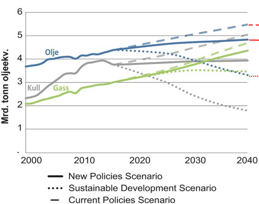
Forbruk av fossile brensler i IEAs scenarier
