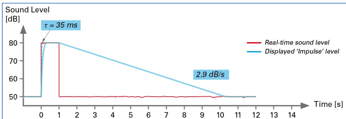
Figur 2-2: Lydtryknivå som funksjon av tiden ved akustisk måling med tidskonstant «Impulse» benyttet i T1442/2012. (Illustrasjon fra NTI-audio) Merk at skalaen er i sekunder. Rød kurve viser det kortvarige målesignalet.
