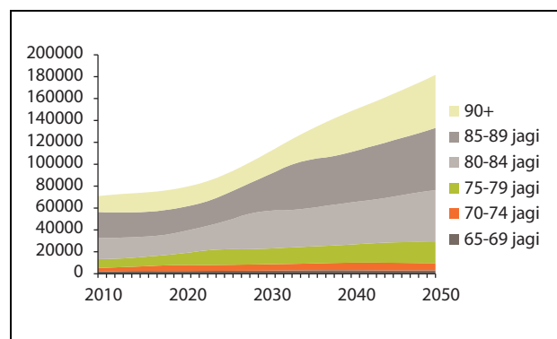
Govus 3.14 Demeanta olbmuid ovddalgihtii árvvoštallojuvvon lohku 2010–2050
