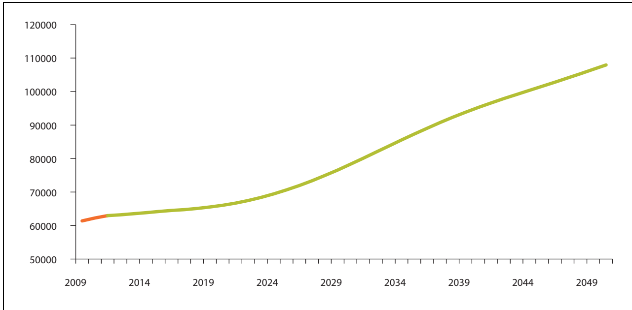
Govus 3.24 Ollesjándora fuolahansajiid ovddalgihtii árvvoštallan 2012–2050
